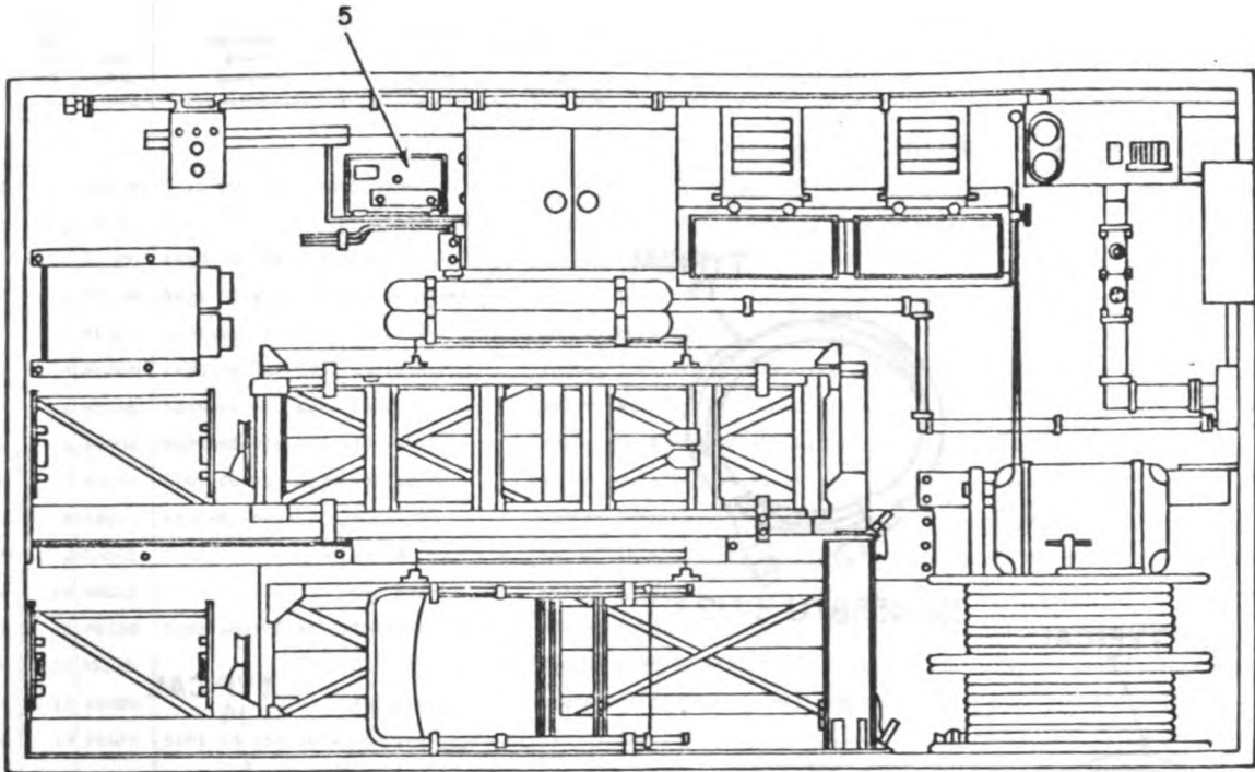
CURBSIDE WALL
