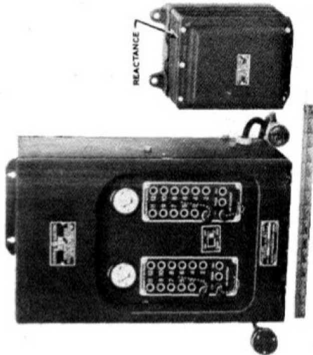
FIGURE 1236. Rectifier RA-36-1 ( )
